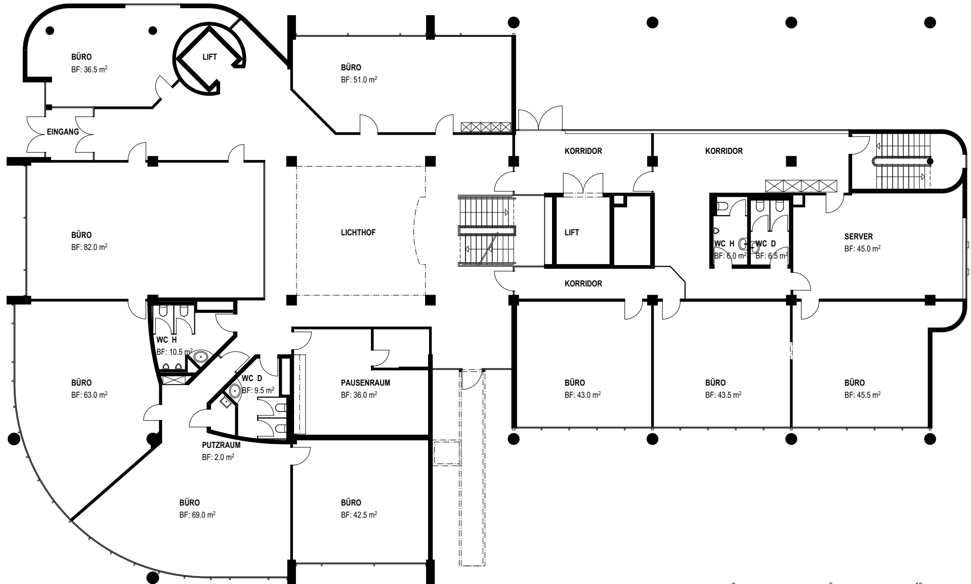
ERDGESCHOSS
